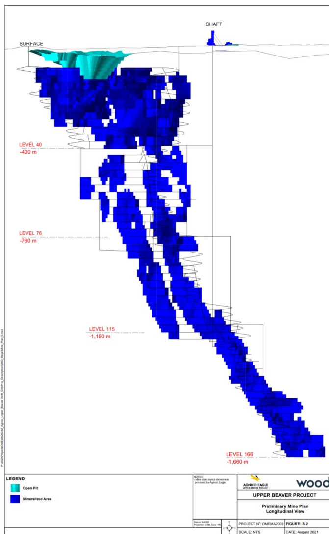
Figure 1. Coupe transversale du projet Upper Beaver montrant la fosse à ciel ouvert, les chantiers souterrains, les rampes d'accès et le puits permettant l'accès au gisement
