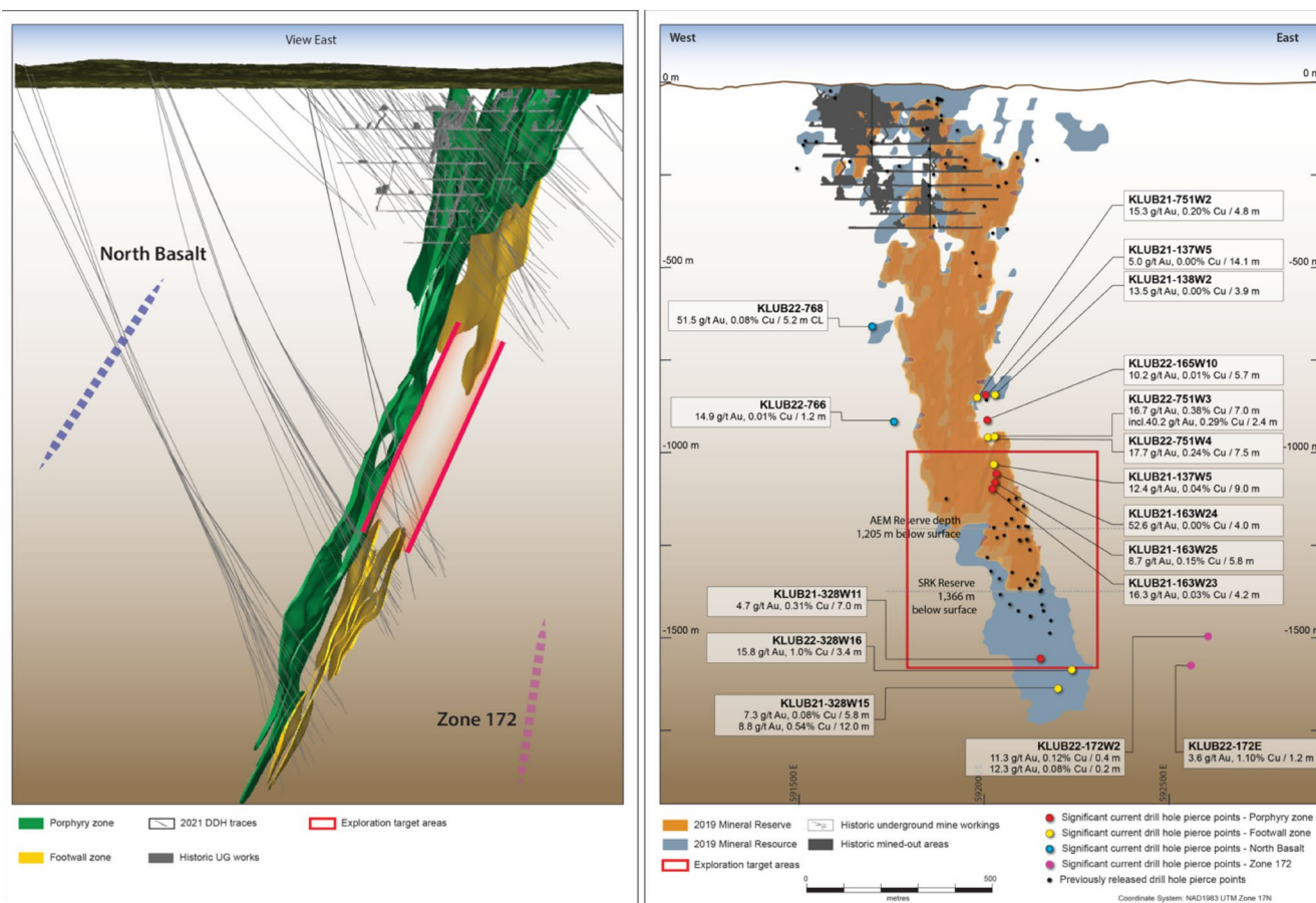
Figure 5 : coupe longitudinale du gisement Upper Beaver
