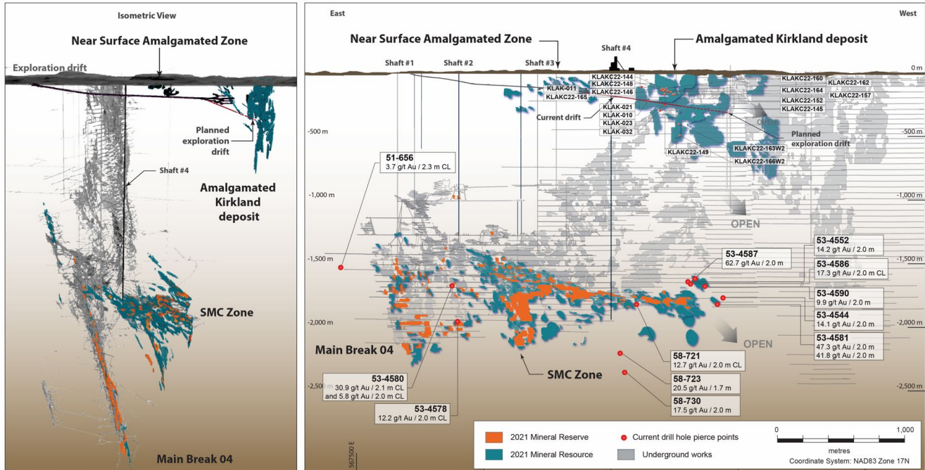
Figure 3 : coupe longitudinale de la mine Macassa et du gisement AK
