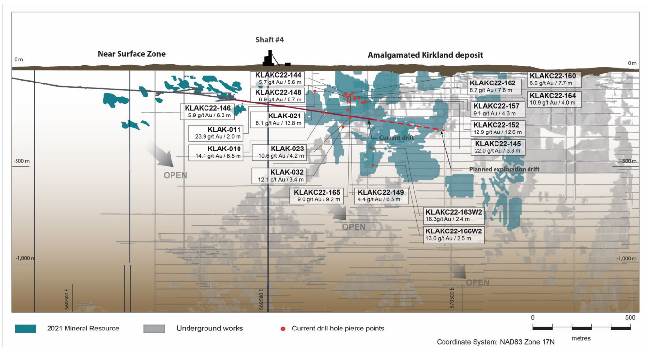
Figure 4 : coupe longitudinale du gisement AK
