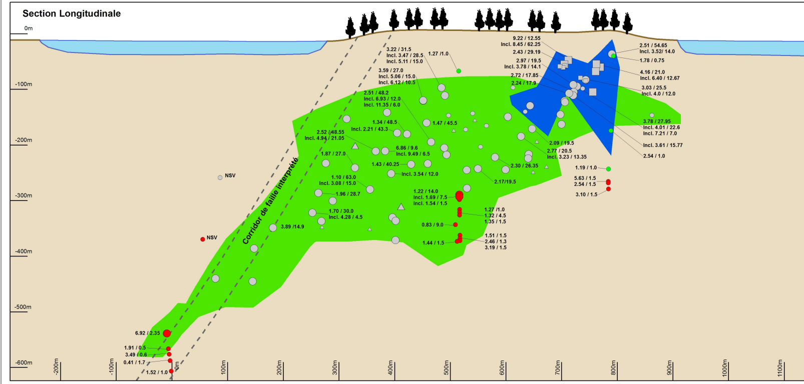
0 25 50 100 Mètres UTM NAD 83 Zone 18 Figure 1 - Section longitudinale Communiqué de presse 6 juin, 2019
